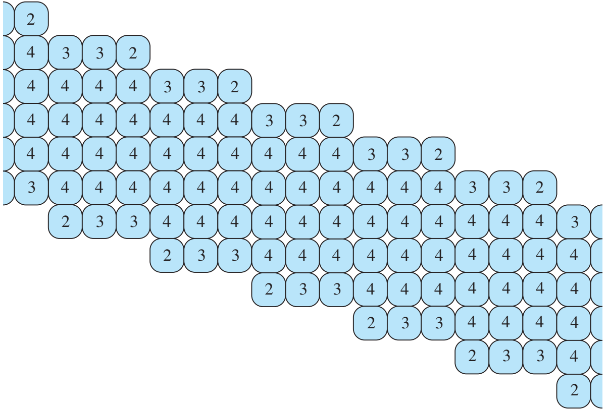
FIG. 1: Cristal bidimensionnel de réseau carré dont la ligne de surface se compose de terrasses avec n = 3 atomes suivies de marches avec un atome.
